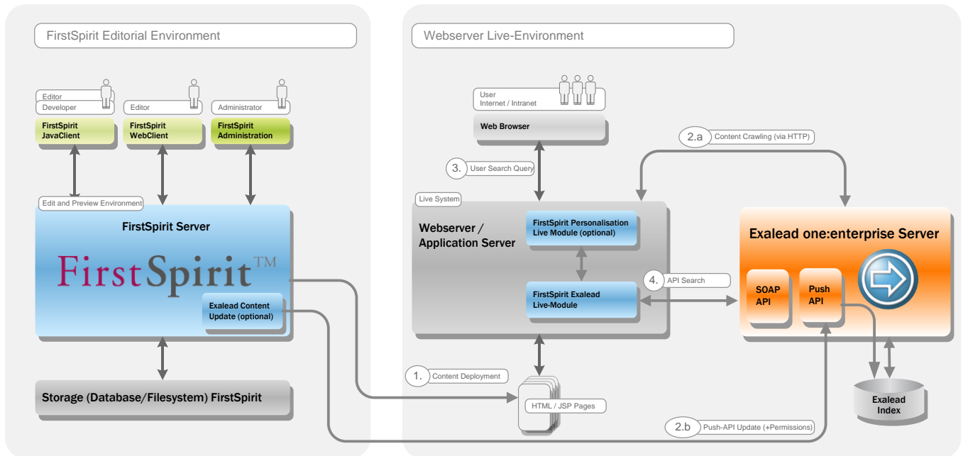
Abbildung 2-3: Push-API-Architektur
