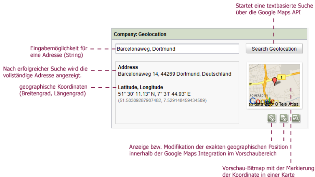
Abbildung 4-6: Geolocation-Eingabekomponente
