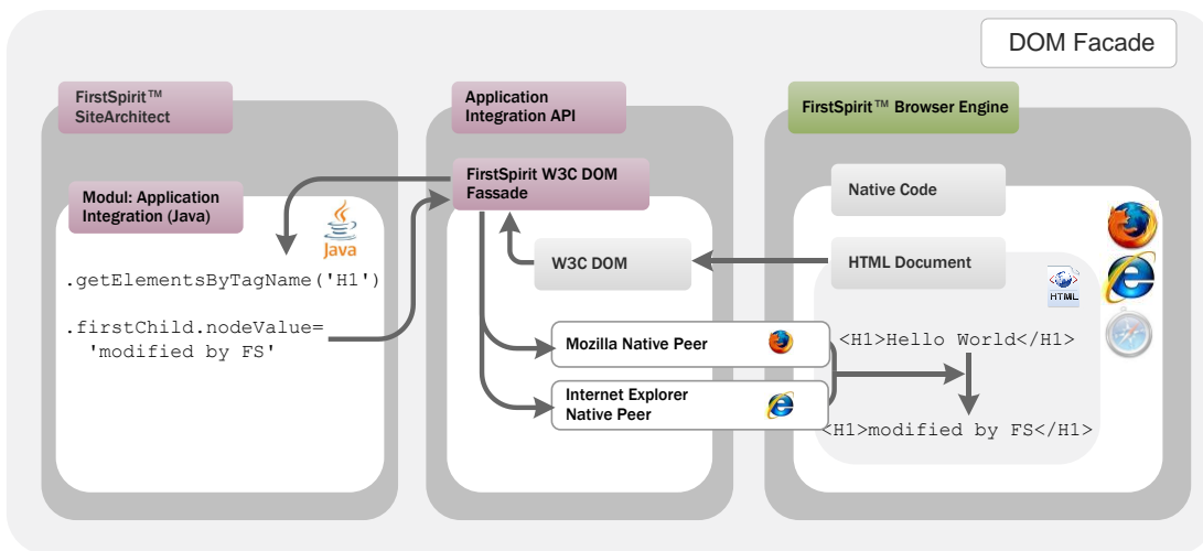
Abbildung 2-2: DOM-Access
