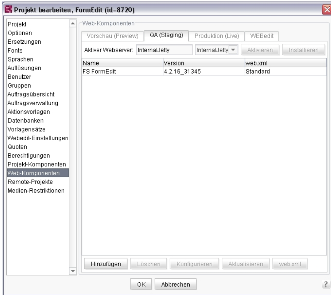
Abbildung 2-4: Installation der Webanwendung innerhalb der Web-Bereiche
