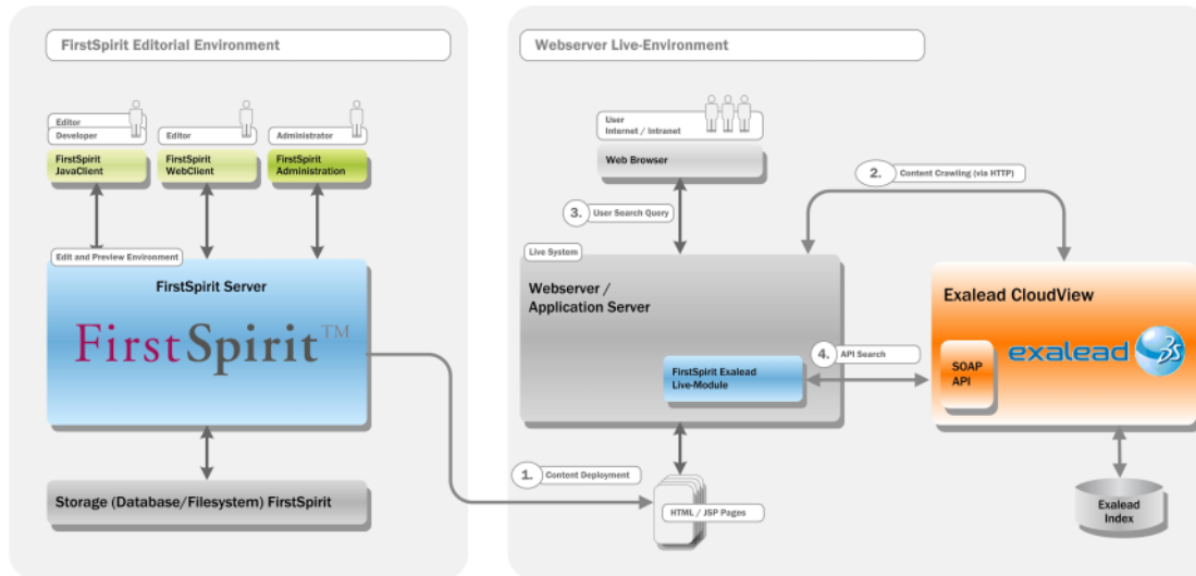
Abbildung 2-1: Basisarchitektur
