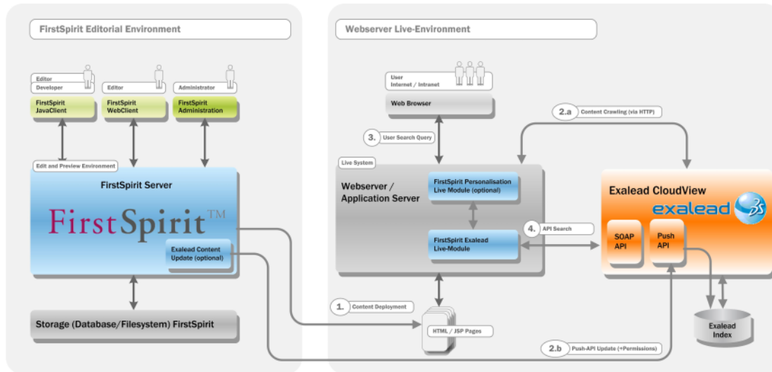
Abbildung 2-3: Push-API-Architektur
