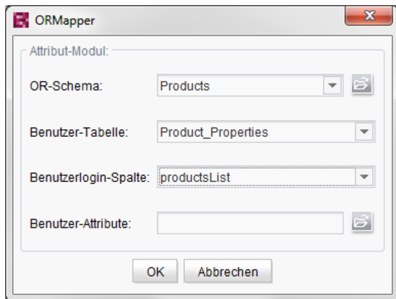
Abbildung 3-15: Attribut-Modul "ORMapper"
