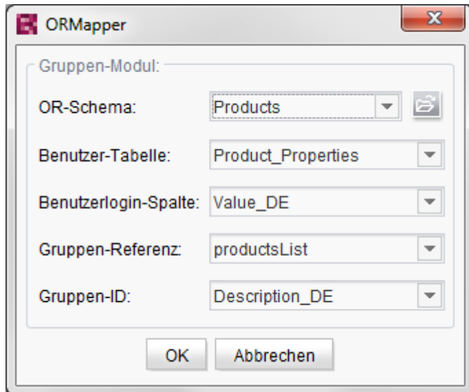
Abbildung 3-12: Gruppen-Modul "ORMapper"
