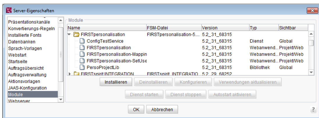
Abbildung 2-1: Installation des Moduls auf dem FirstSpirit-Server
