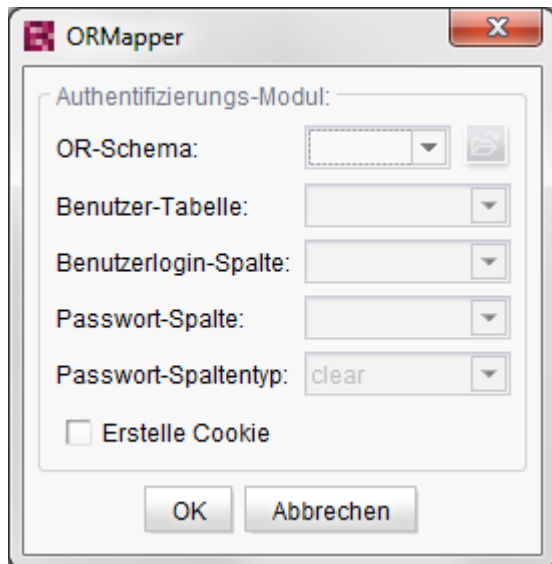
Abbildung 3-6: Authentifizierungs-Modul "ORMapper"
