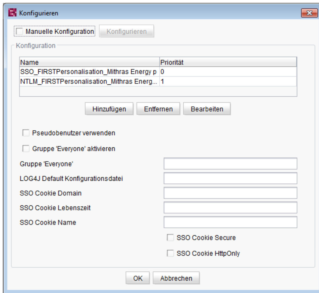
Abbildung 2-4: Konfigurieren der Webanwendung Integration
